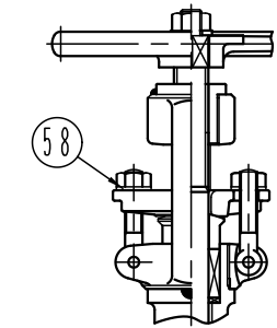
40A(11/2B), 50A(2B) DETAIL
